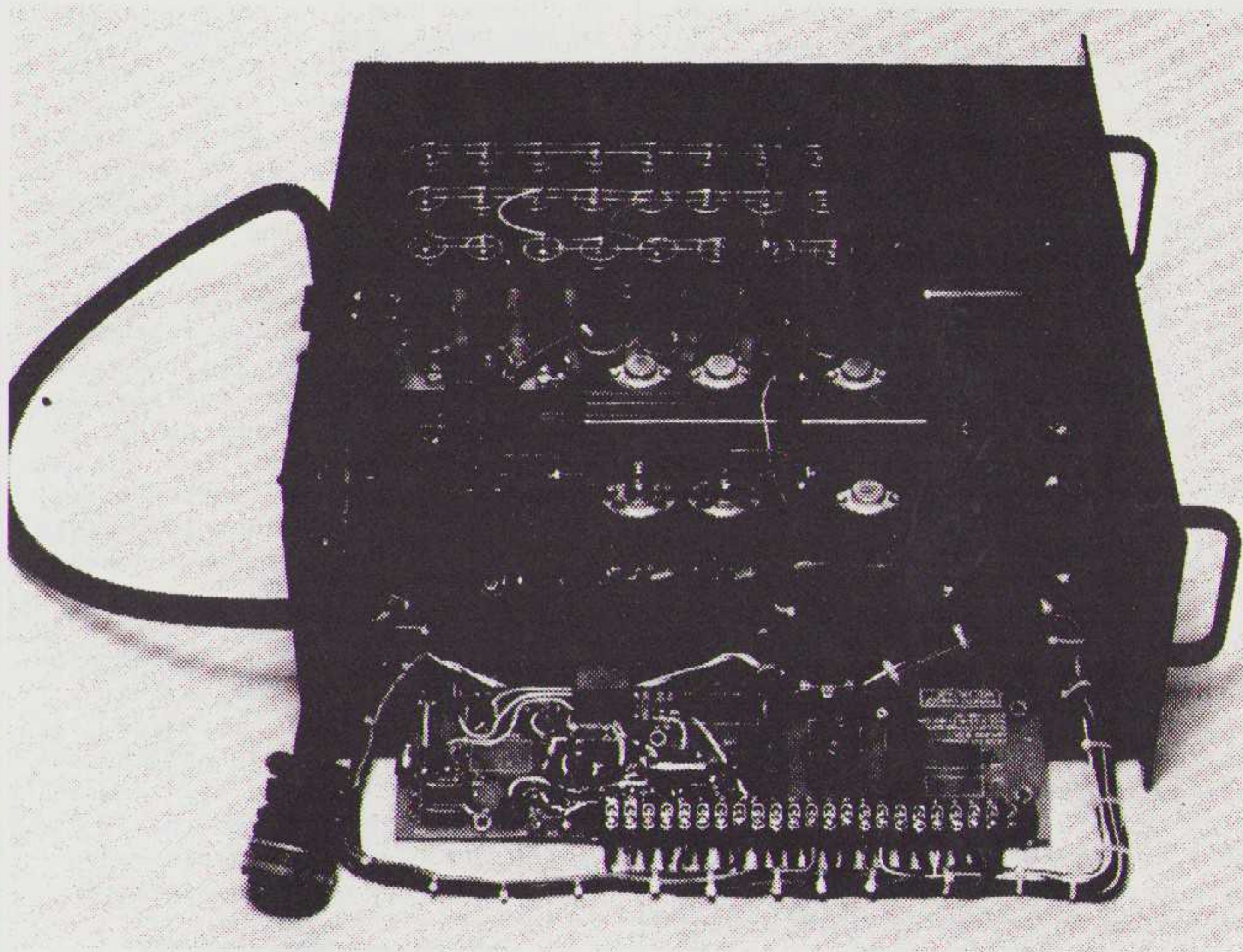
Gestabiliseerde voeding 350 V 510 A voor de versterker OTL-1 van Futterman
